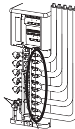
Raccordement de l'écrou évasé (Unité extérieure)
