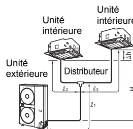
Figure de l'installation double simultanée
