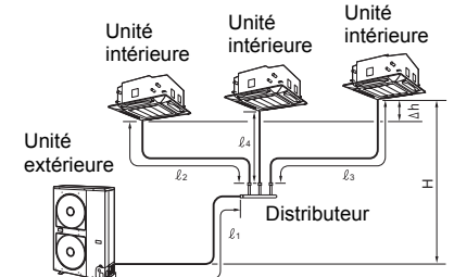
Figure de l'installation triple simultanée
